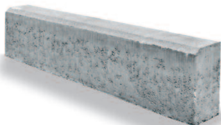
Kiemelt útszegély kopóréteggel Méret: 100 x 25 x 8 cm Szín: szürke
