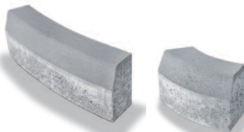
Íves útszegélyek Méretek: 39 x 25 x 15 cm, R = 0,5 m 52 x 25 x 15 cm, R = 1,0 m 78 x 25 x 15 cm, R = 2,0 m 78 x 25 x 15 cm, R = 3,0 m Szín: szürke
