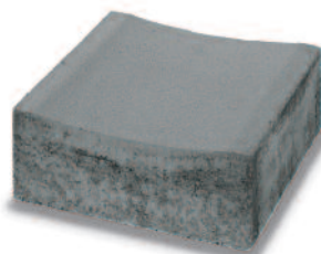
Betonfolyóka 1,5 cm horonymélységgel Méret: 40 x 40 x 8 cm Szín: szürke
